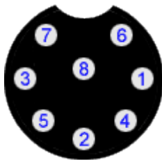
8 Pin DIN DIN 45326
