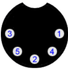
5 Pin DIN DIN 41524
